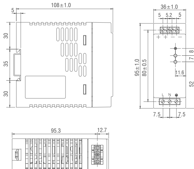
BPS-1-30-12DC & BPS-1-30-24DC
