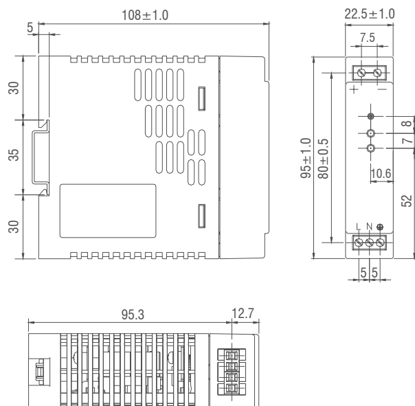
BPS-1-15-12DC & BPS-1-15-24DC
