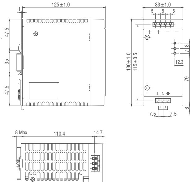
BPS-1-70-12DC & BPS-1-70-24DC
