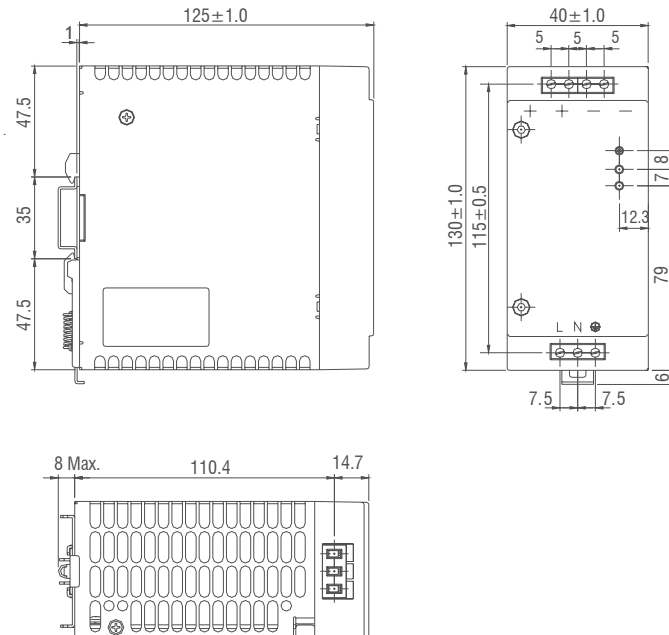
BPS-1-120-12DC & BPS-1-120-24DC
