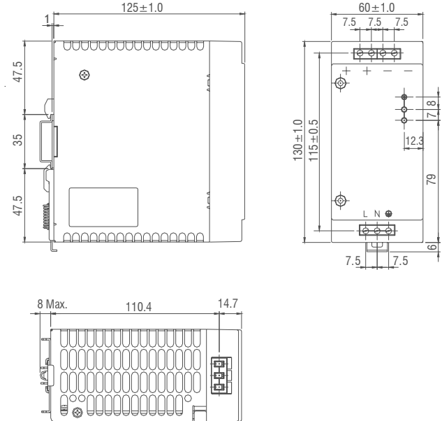
BPS-1-240-24DC
